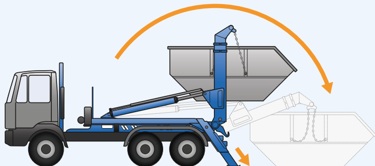
Odstavení kontejneru ...
